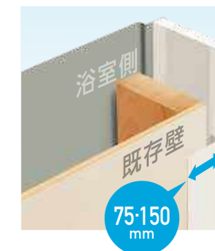
抗菌樹脂枠 隙間化粧カバー L字タイプ
